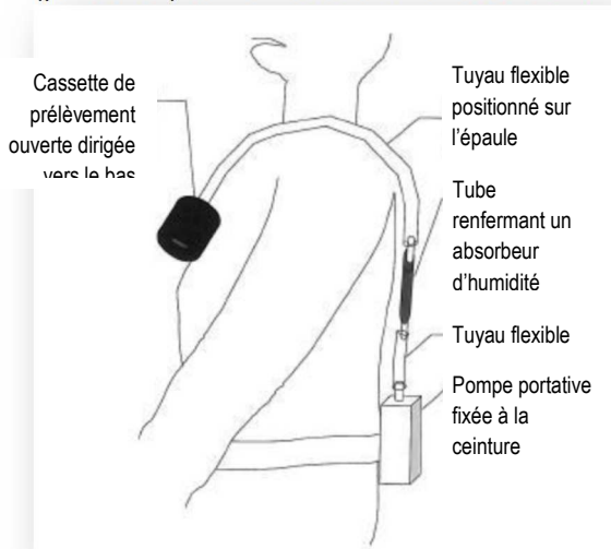
Schéma de la pose d'une pompe sur compagnon
