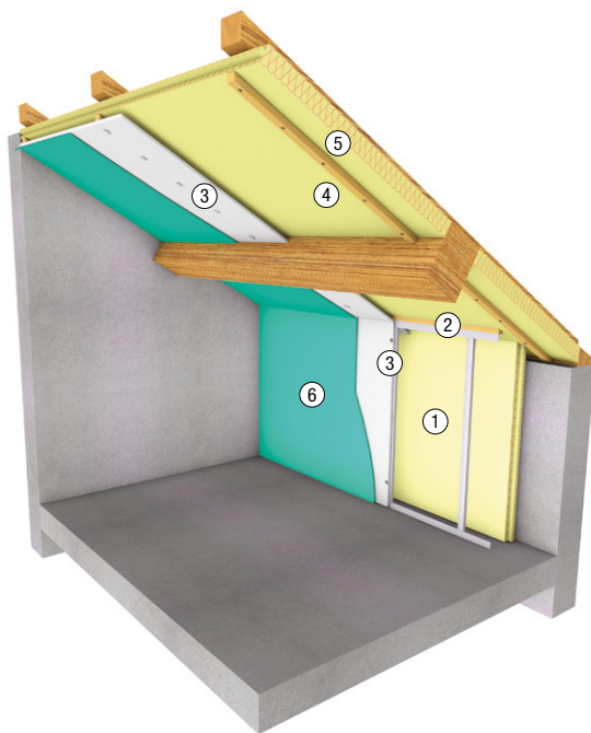
Schéma N°10 Isolation comble aménageable sous chevron
