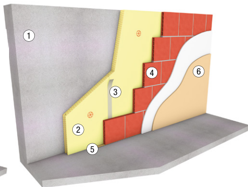
Schéma N°3 Contre-cloison maçonnerie
