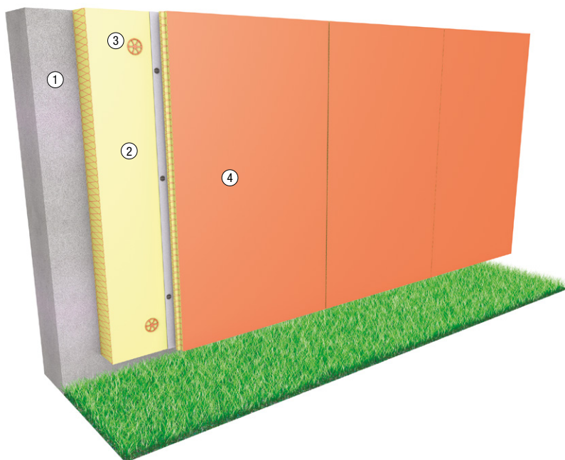
Schéma N°15 Isolant PU sous Vêture PU
