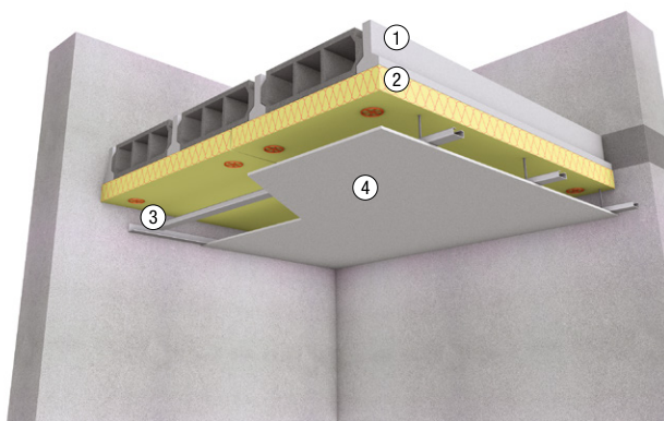
Schéma N°6 Isolation sous plancher
