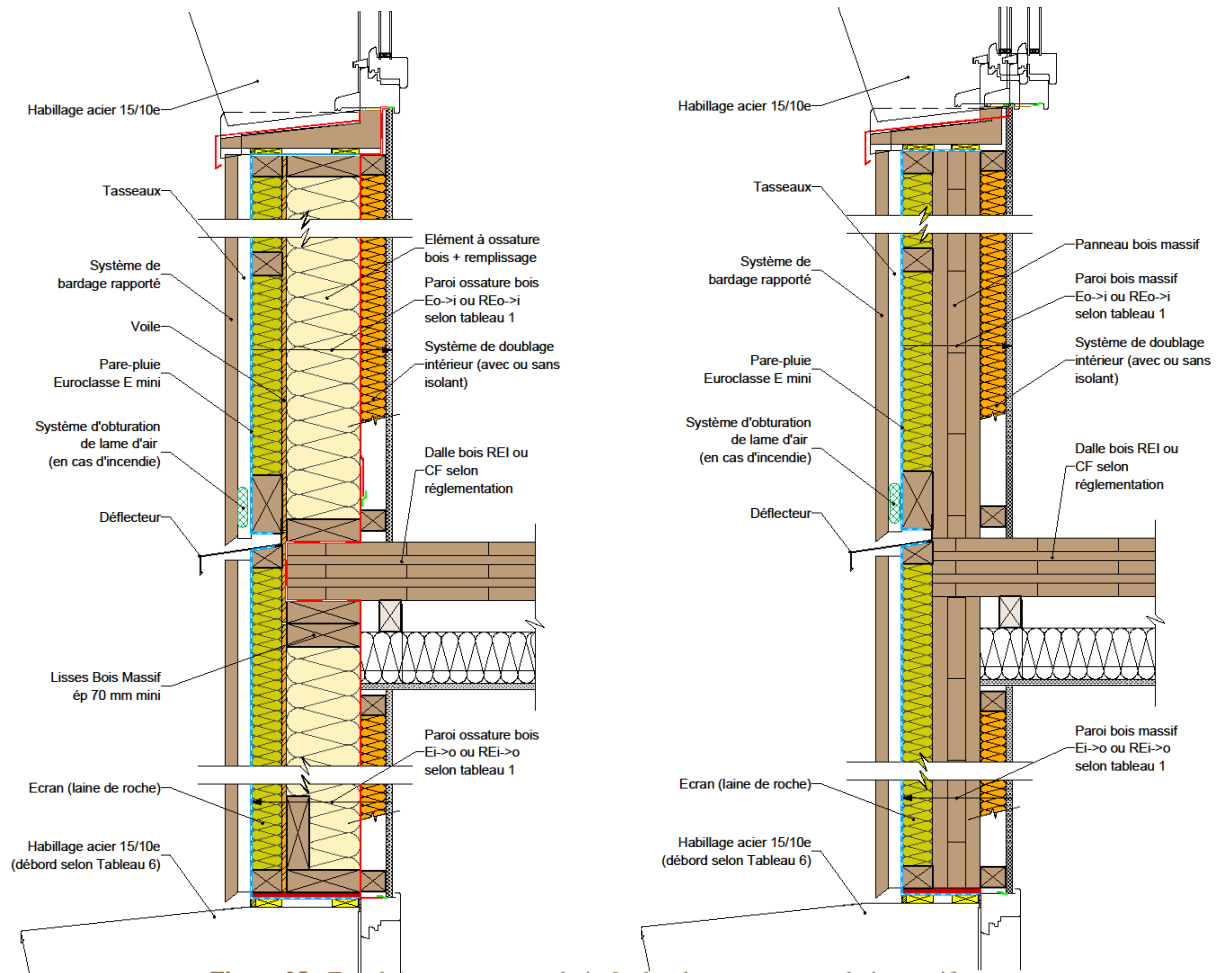
Figure 25 : Façade/mur en ossature bois & plancher en panneaux bois massif.
