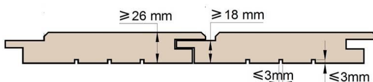
Figure 7: Epaisseurs des profils de bardage – Prescriptions.
