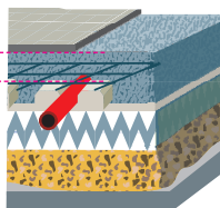
Plancher de type A (cf p8)
