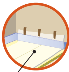
Jointolement par un film de protection en polyéthylène de 0,15 mm (150 μm) d'épaisseur minimale
