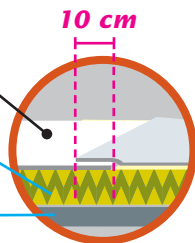
Jointolement par un film de protection en polyéthylène de 0,15 mm (150 μm) d'épaisseur minimale
