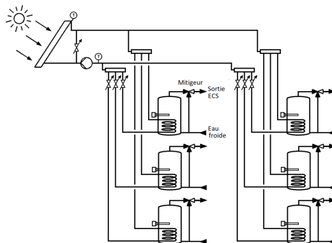
Figure 73 Chauffe-eau solaires collectifs individualisés (CESCI)
