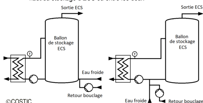
Figure 35 Raccordements du retour de bouclage et de l'arrivée d'eau froide visés
