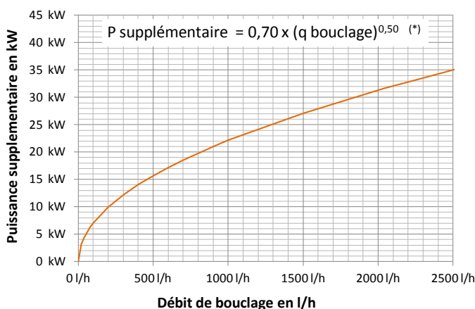
Figure 36 Puissance supplémentaire requise pour le bouclage dans le cas d'un raccordement du retour de boucle et de l'arrivée d'eau froide en bas du stockage ECS
