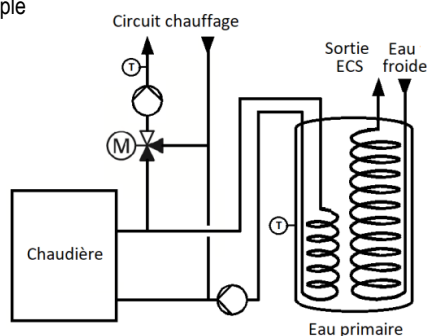
Figure 57 Ballon de stockage d'eau primaire, raccordé via un échangeur à la chaudière, doté d'un échangeur immergé pour la production d'ECS
