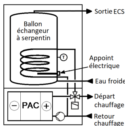
Figure 16 Pompes à chaleur double-service
