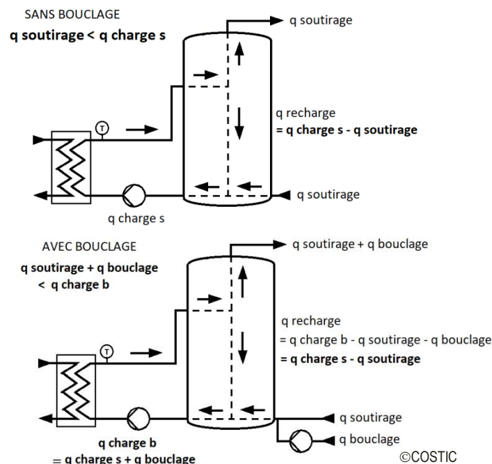
Figure 41 Impact du débit de retour de bouclage durant la recharge du stockage
