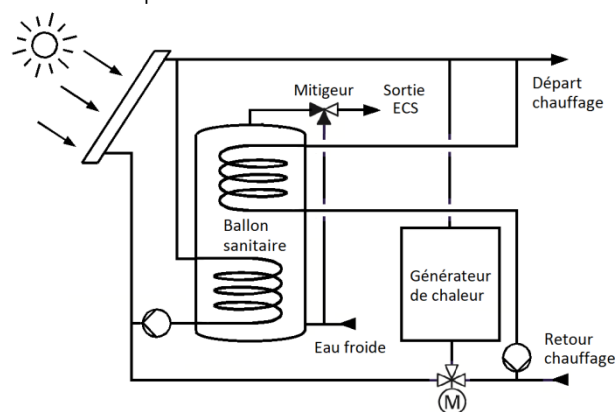
Figure 14 Système solaire combiné
