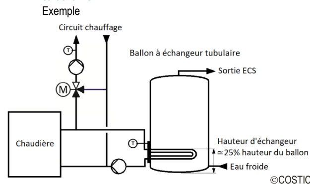
Figure 44 Production d'ECS par un ballon à échangeur tubulaire
