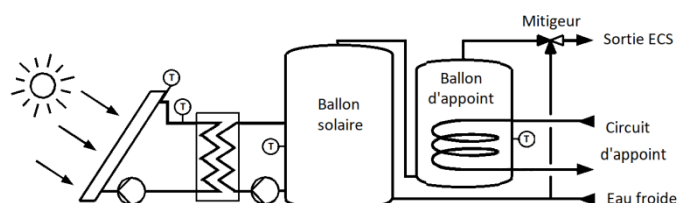
Figure 72 Chauffe solaire centralisé avec un stockage en eau primaire
