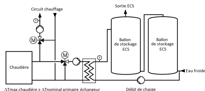
Figure 21 Production par échangeur et ballons d'ECS avec une circulation continue
