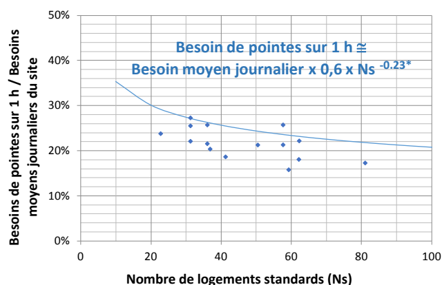
Figure 19 Pourcentages des besoins moyens journaliers correspondant aux besoins de pointes sur 1 h Résultats obtenus pour 21 sites ayant fait l'objet de télésondages.
