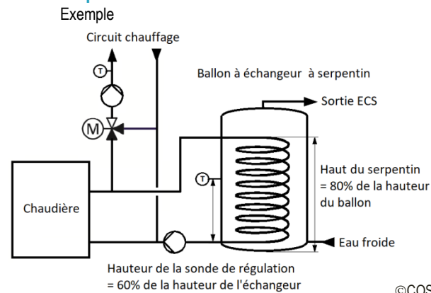
Figure 44 Production d'ECS par un ballon à échangeur tubulaire
