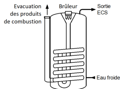
Figure 58 Accumulateur gaz à serpentin
