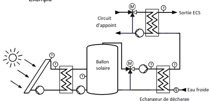
Figure 72 Chauffe solaire centralisé avec un stockage en eau primaire
