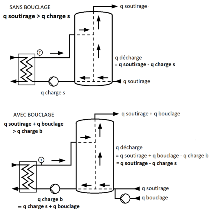
Figure 42 Autres configurations de raccordement lors d'un fonctionnement en décharge durant la pointe maximale de soutirages
