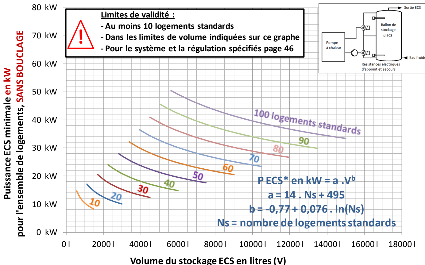
Figure 63 Puissance ECS minimale requise en kW, en fonction du volume de stockage, en litres, pour le système de production par PAC à échange direct avec un stockage ECS « à stratification dynamique »
