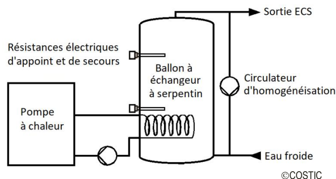
Figure 67 PAC couplée à un ballon à échangeur avec un appoint électrique dans le ballon et un circulateur d'homogénéisation
