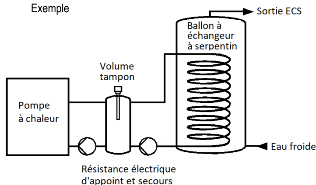
Figure 66 PAC couplée à un ballon à échangeur avec un appoint électrique intégré dans le volume tampon de la PAC
