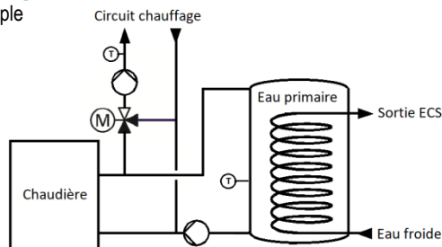
Figure 57 Ballon de stockage d'eau primaire, raccordé via un échangeur à la chaudière, doté d'un échangeur immergé pour la production d'ECS
