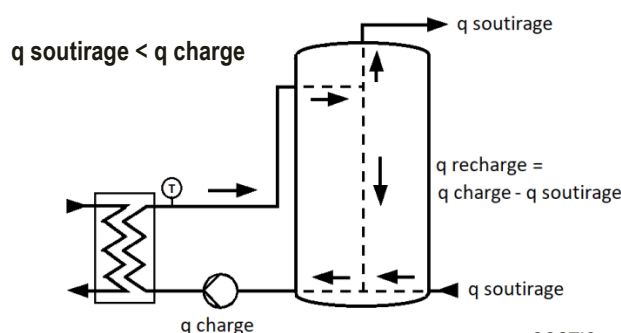
Figure 23 Fonctionnement de ce système pour un débit de soutirage inférieur au débit de charge
