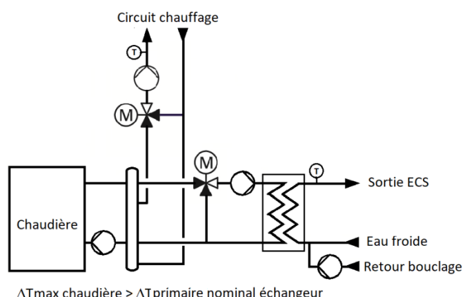
Figure 20 Production collective instantanée d'ECS par échangeur sans stockage
