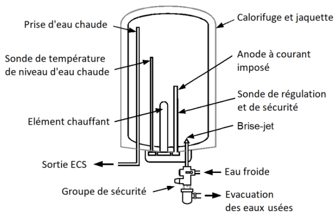
Figure 9 Ballon électrique vertical
