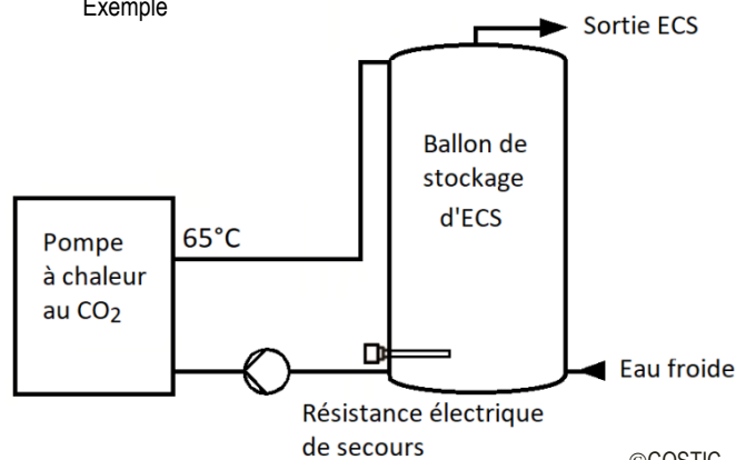
Figure 59 PAC au CO 2 à échange direct couplée à un ballon de stockage d'ECS
