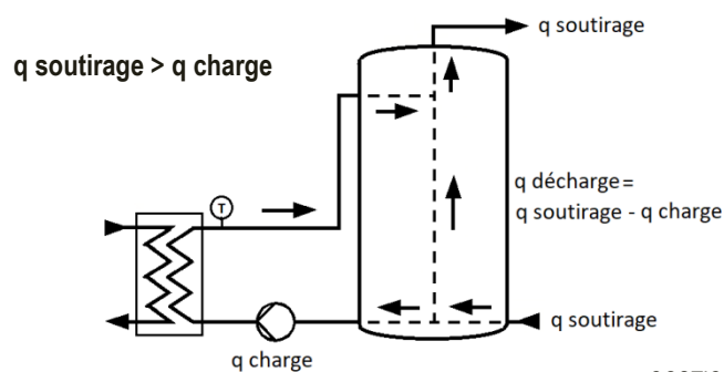
Figure 24 Fonctionnement de ce système pour un débit de soutirage supérieur au débit de charge
