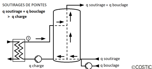
Figure 38 Fonctionnement lors des puisages de pointes
