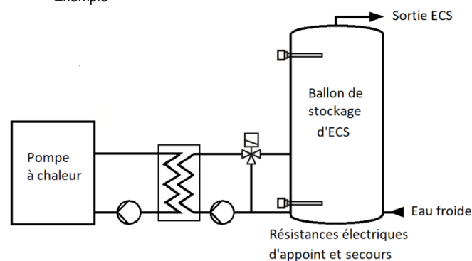
Figure 64 PAC associée à un échangeur externe et des ballons de stockage d'ECS
