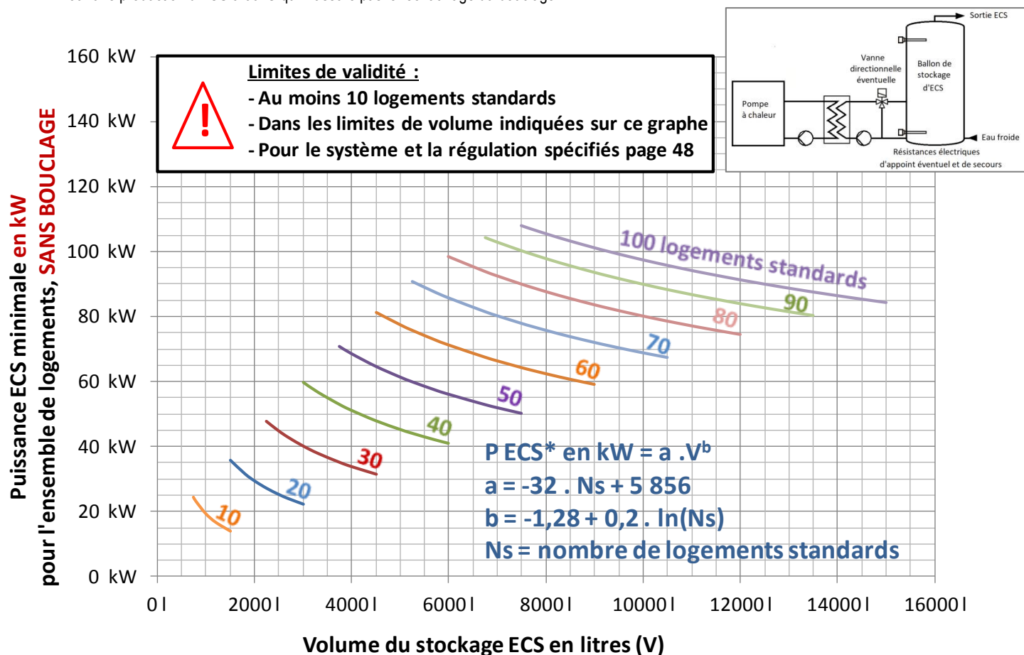
Figure 65 Puissance ECS minimale requise en kW, en fonction du volume de stockage, en litres, pour le système de production par PAC avec échangeur externe associé à un stockage ECS Pour une production d'ECS à 60°C qui n'assure pas le réchauffage du bouclage
