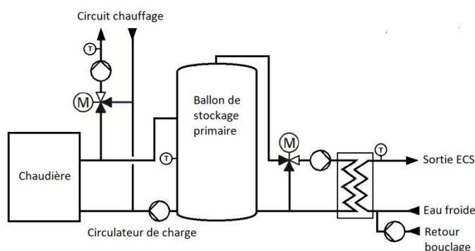
Figure 50 Production collective d'ECS par échangeur et ballon de stockage primaire
