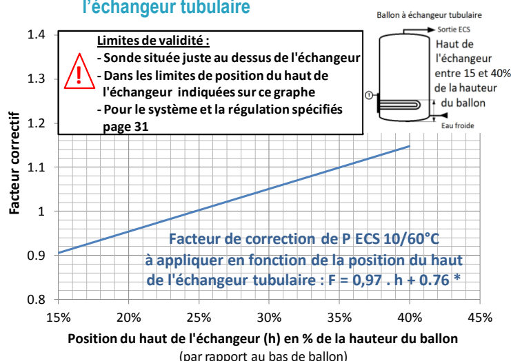
Figure 47 Correction à appliquer aux valeurs de puissance ECS en fonction de la position du haut de l'échangeur tubulaire
