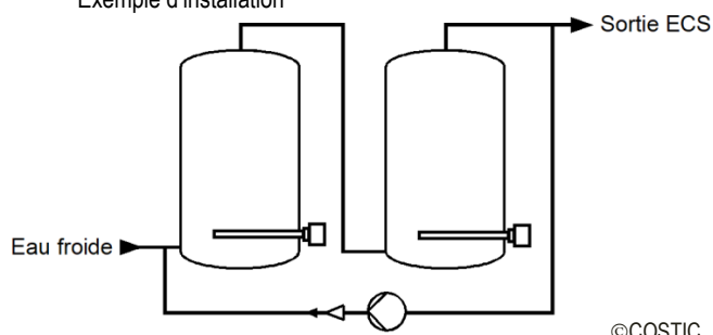
Figure 69 Production collective d'ECS par ballons électriques
