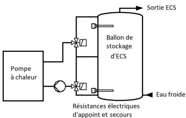
Figure 62 PAC à échange direct avec un stockage d'ECS à « stratification dynamique »
