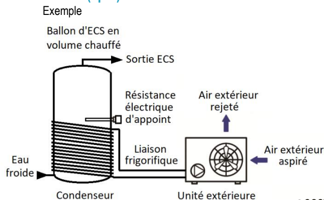
Figure 15 Chauffe-eau thermodynamiques sur air extérieur bi-bloc (split)
