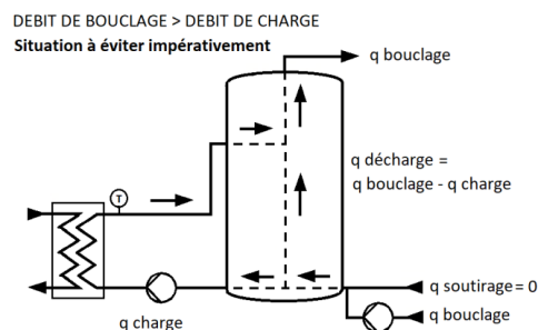
Figure 39 Impact d'un débit de bouclage supérieur au débit de charge
