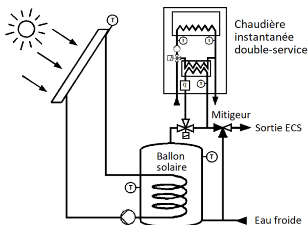
Figure 11 Chauffe-eau solaire individualisé
