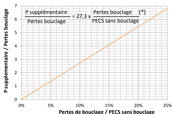
Figure 32 Puissance supplémentaire requise pour le bouclage dans le cas d'un raccordement du retour de bouclage entre le tiers supérieur et le milieu du stockage
