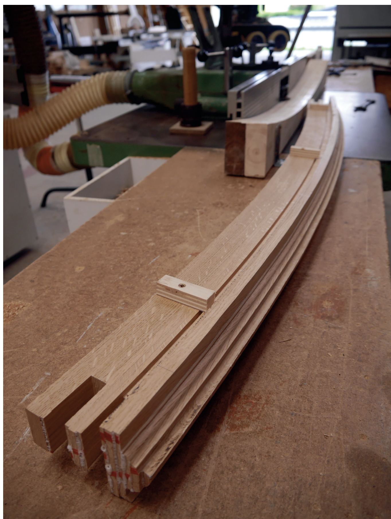
Atelier de l'entreprise Option Bois à Pont Hébert (50) Au premier plan : Traverse basse de l'imposte en cours d'usinage à la toupie. Au second plan : Montage d'usinage permettant les profilages sur les pièces cintrées.
