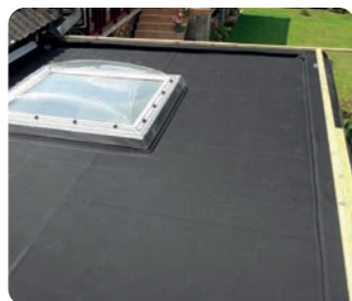
Membranes EPDM
